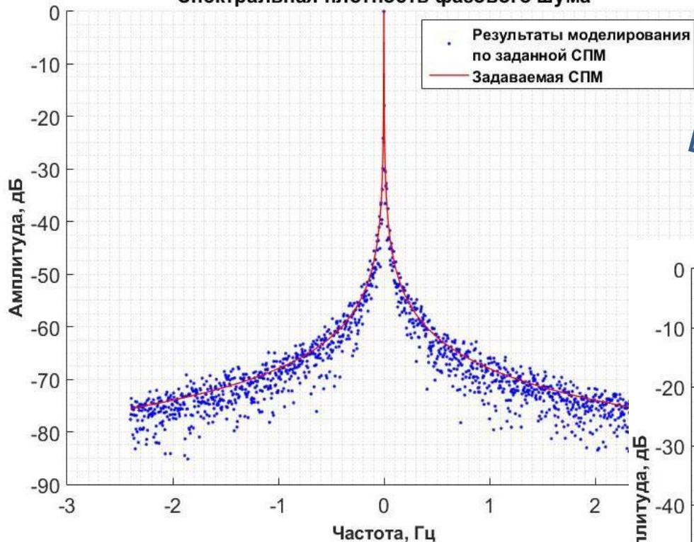
Спектральная плотность фазового шума
