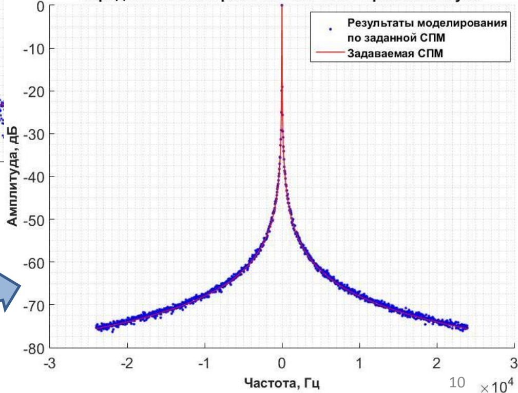
Усредненная спектральная плотность фазового шума
